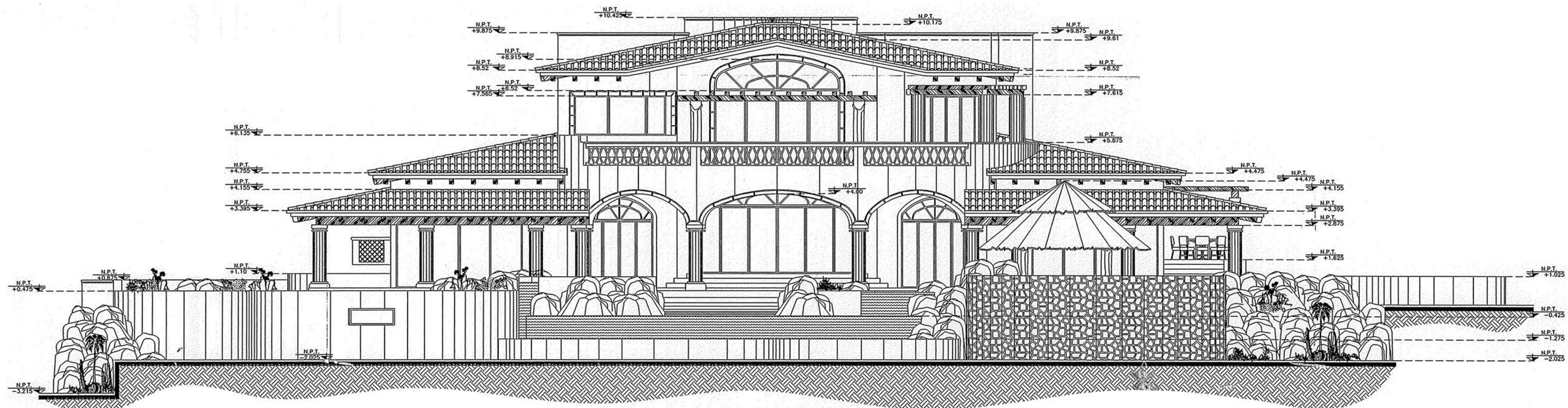
02 FACHADA POSTERIOR 1:75
